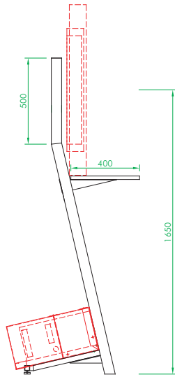
SEITENANSICHT BOXPOSITION 2
