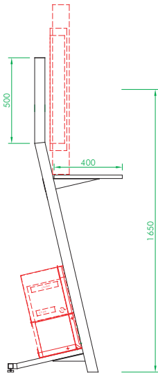
SEITENANSICHT BOXPOSITION 1
